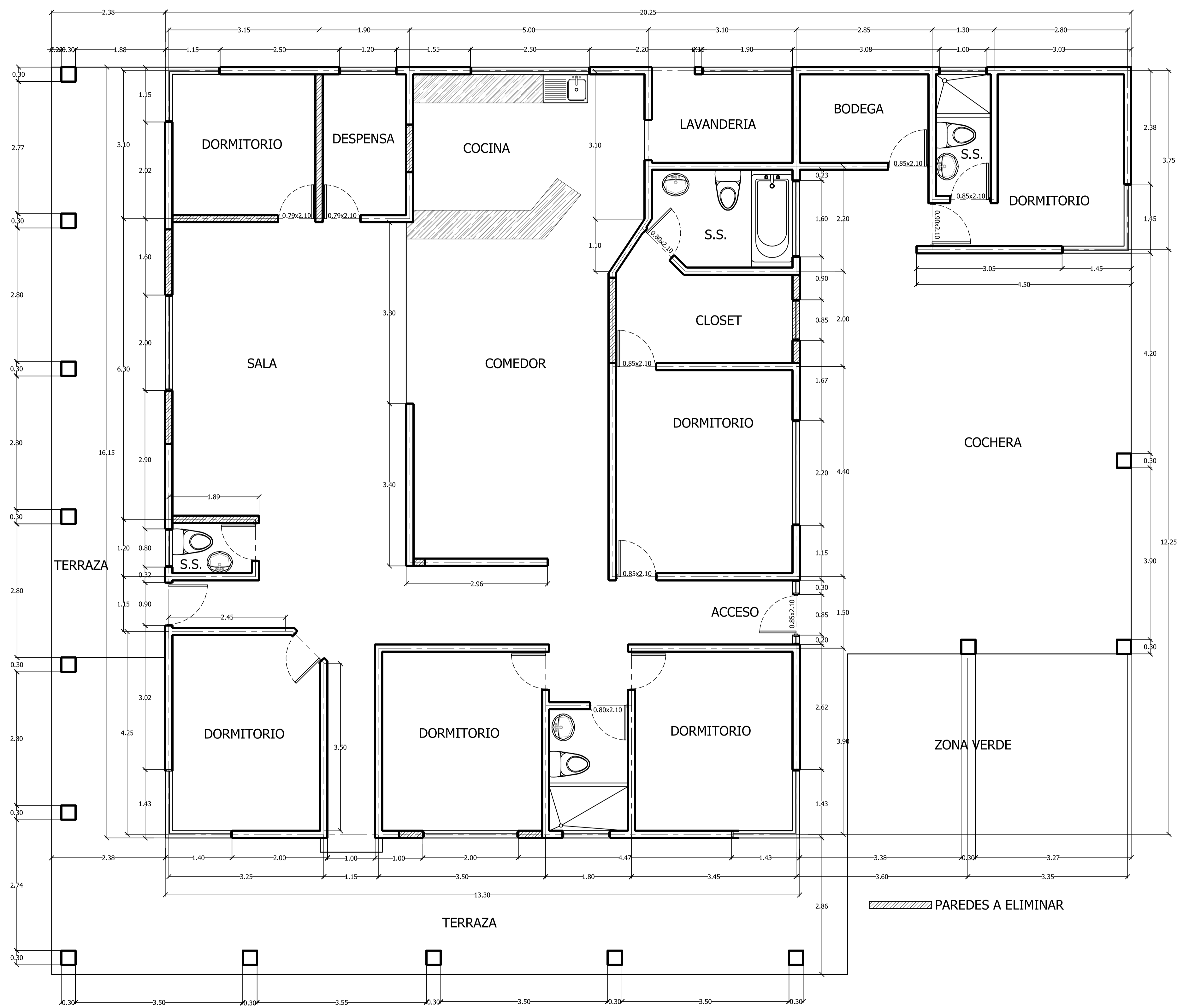
PLANTA DISTRIBUCION ARQUITECTONICA EXISTENTE ESCALA 1:50
